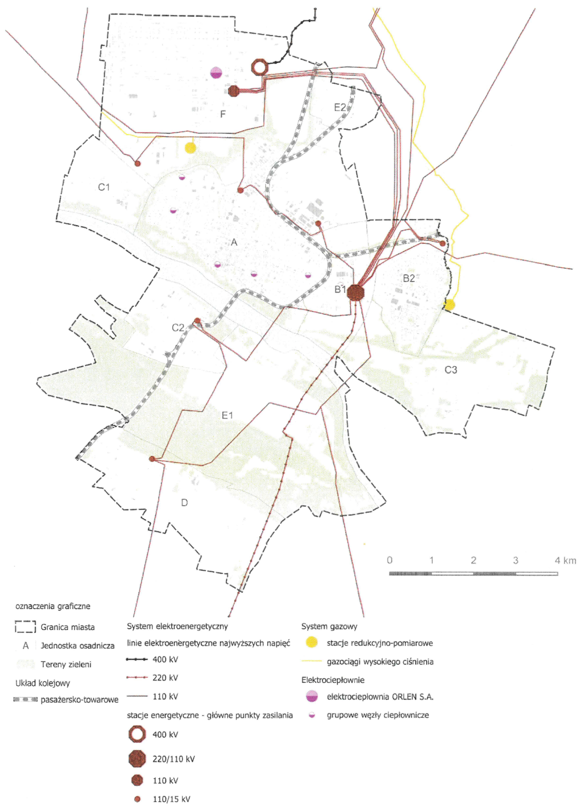
Grafika 13 Mapa infrastruktury technicznej: system elektroenergetyczny, system gazowy, elektrociepłownie
