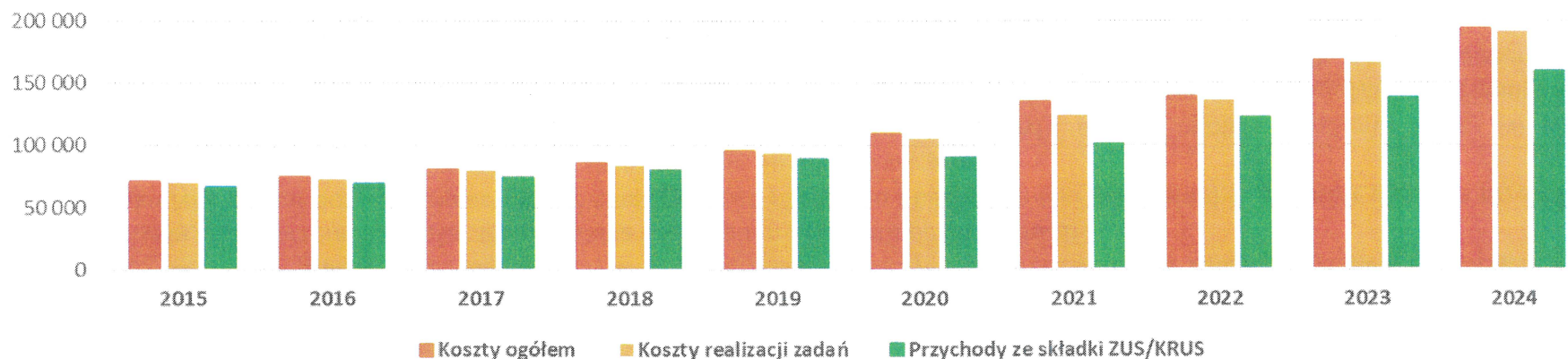
Koszty NFZ vs. przychody ze składek ZUS/KRUS w latach 2015-2024 w mld zł.
